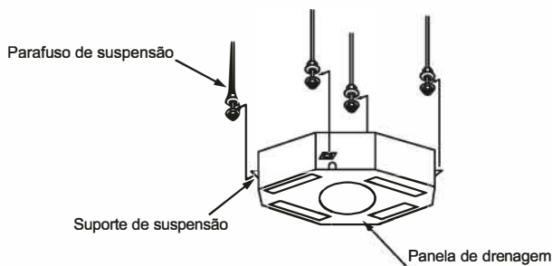
Fig.3.8 Montagem da Unidade Interior
