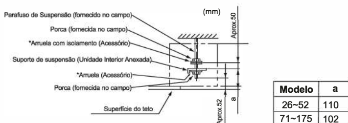
Fig.3.7 Montagem Porcas e arruela
