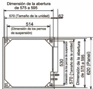
Imagen 3.3 Abertura del falso techo y pernos de suspensión
