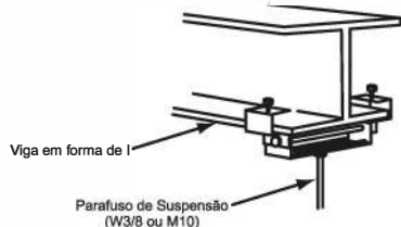
Fig. 3.4 Montagem dos Parafusos de Suspensão
