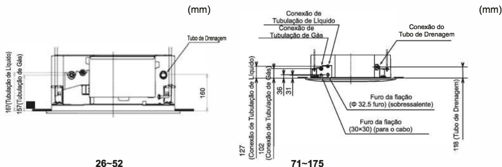
Fig.3.6 Unidade Interior e Pannel de Ar
