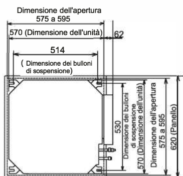
Fig. 3.3. Apertura del controsoffitto e bulloni di sospensione
