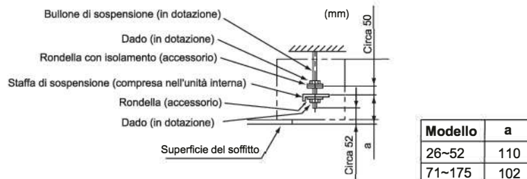
Fig.3.7 Montaggio dei dadi e della rondella
