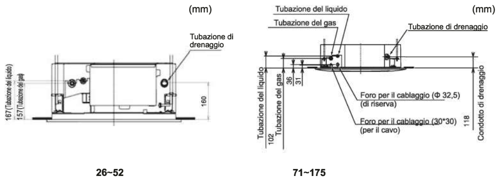
Fig 3.6 Unità interna e pannello dell'aria
