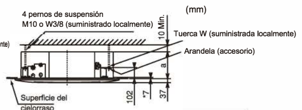
Imagen 3.4 Montaje de los pernos de suspensión
