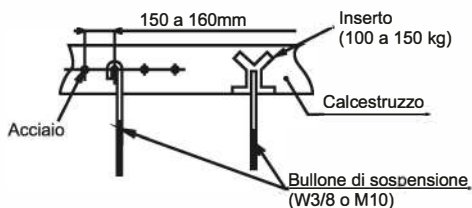
Fig. 3.4. Montaggio dei bulloni di sospensione
