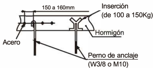
Imagen 3.4 Montaje de los pernos de suspensión
