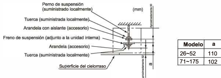
Imagen 3.7 Montaje de las tuercas y arandela
