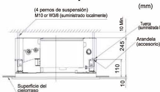
Imagen 3.5 Posición de montaje
