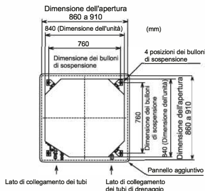
Fig. 3.3. Apertura del controsoffitto e bulloni di sospensione
