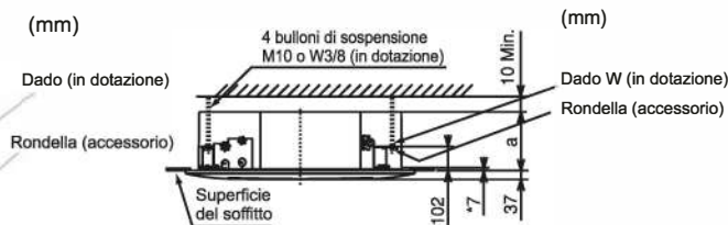
Fig. 3.4. Montaggio dei bulloni di sospensione
