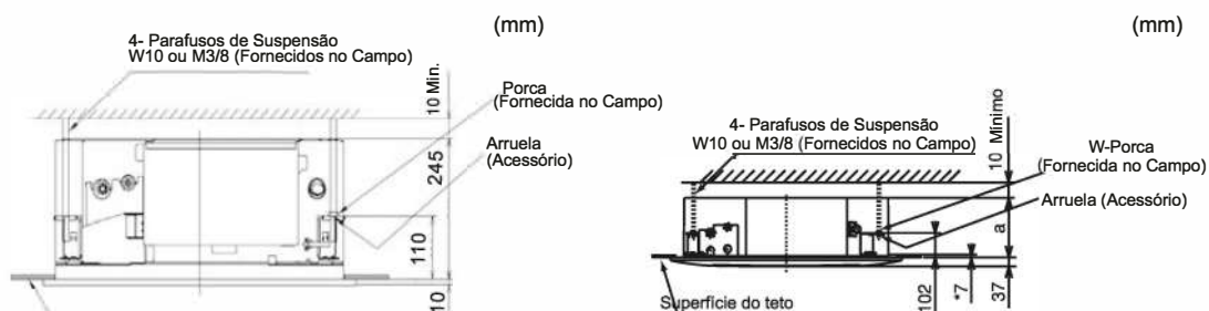
Fig. 3.4 Montagem dos Parafusos de Suspensão
