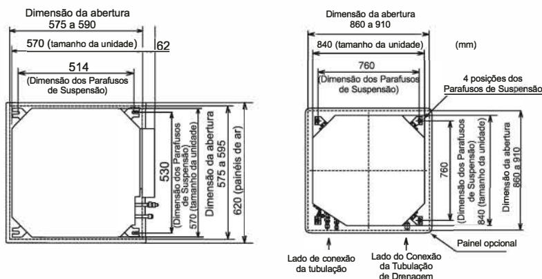
Fig 3.3 Abertura de Teto Falso e Parafusos de Suspensão
