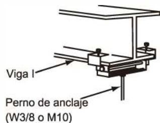
Imagen 3.4 Montaje de los pernos de suspensión
