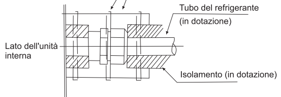
Fig 4.4 Procedura di isolamento dei tubi
