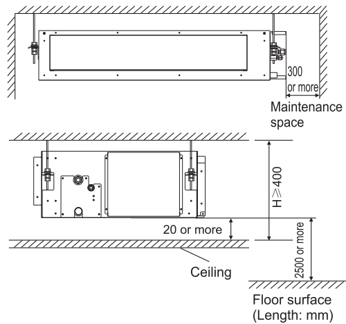
Fig. 3.1.2 (unit: mm)
