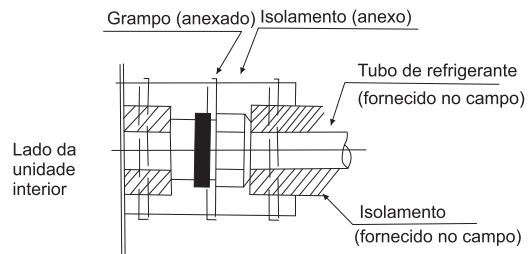
Fig. 4.4 Procedimento de isolamento da tubagem
