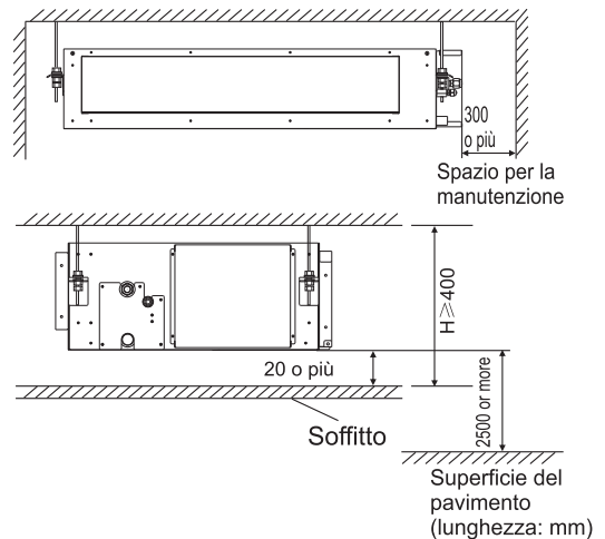
Fig. 3.1.2 (Unità: mm)
