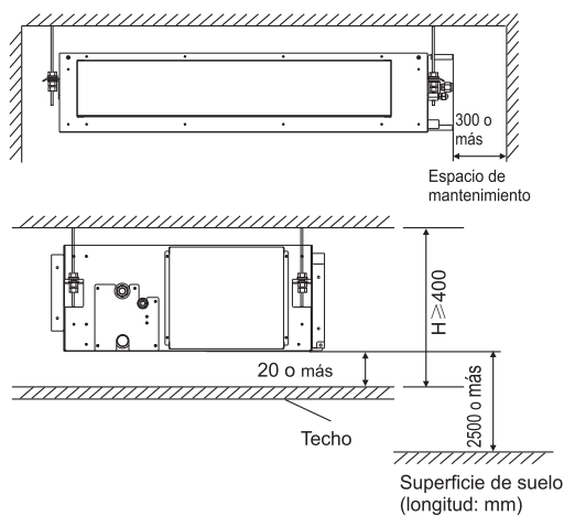
Fig. 3.1.2 (unit: mm)
