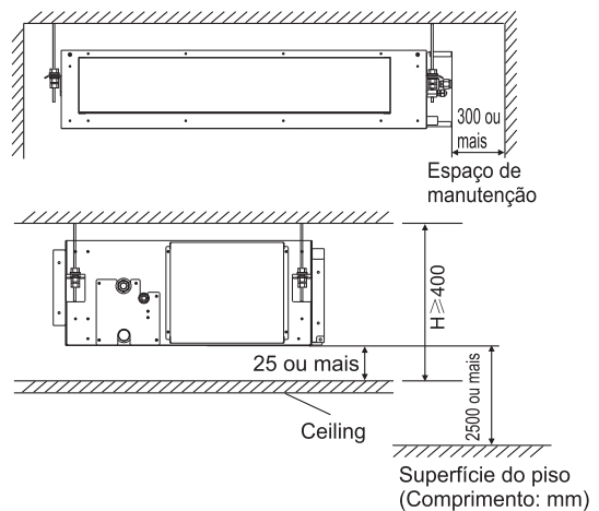
Fig. 3.1.2 (unidade: mm)
