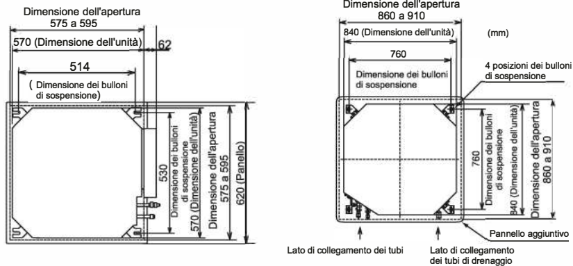
Fig. 3.3. Apertura del controsoffitto e bulloni di sospensione
