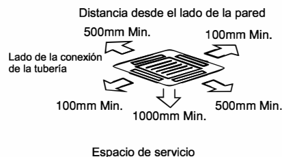
Imagen 3.1 Espacio alrededor de la unidad interna
