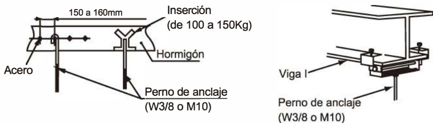
Imagen 3.4 Montaje de los pernos de suspensión
