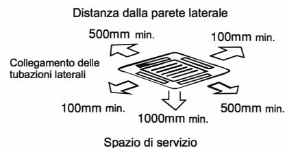
Fig. 3.1 Spazio intorno all'unità interna
