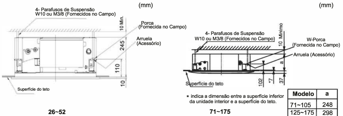
Fig.3.5 Posição de Montagem
