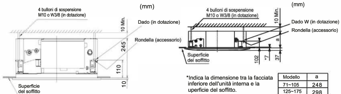
Fig.3.5 Posizionamento
