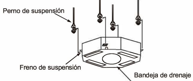
Imagen 3.8 Montaje de la unidad interna
